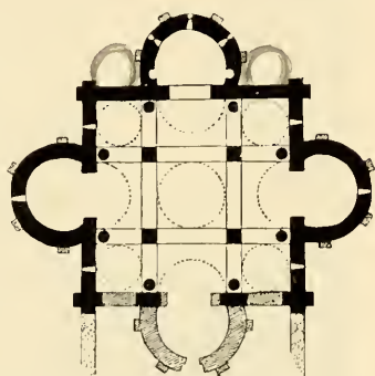
■ Parti della basilica primitiva tuttora esistenti - - - Parti state sopresse □ Parti aggiunte nel sec. XI
